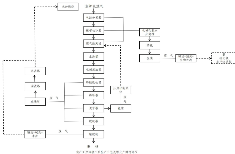
图 3-6 化产工序回收二系生产工艺流程及产排污图
