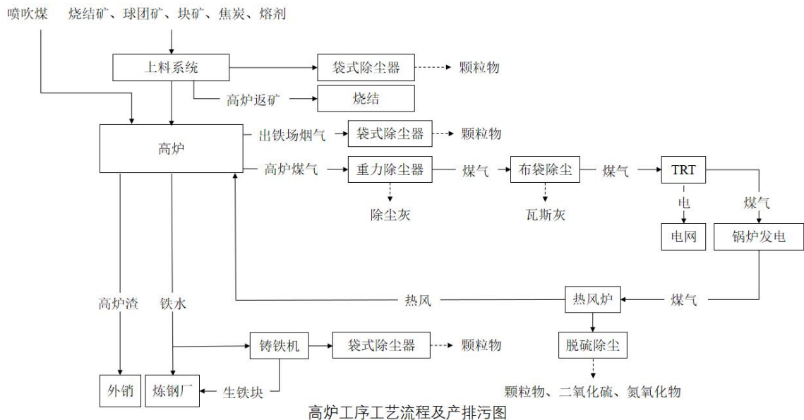
图 3-7 高炉工序工艺流程及产排污图
