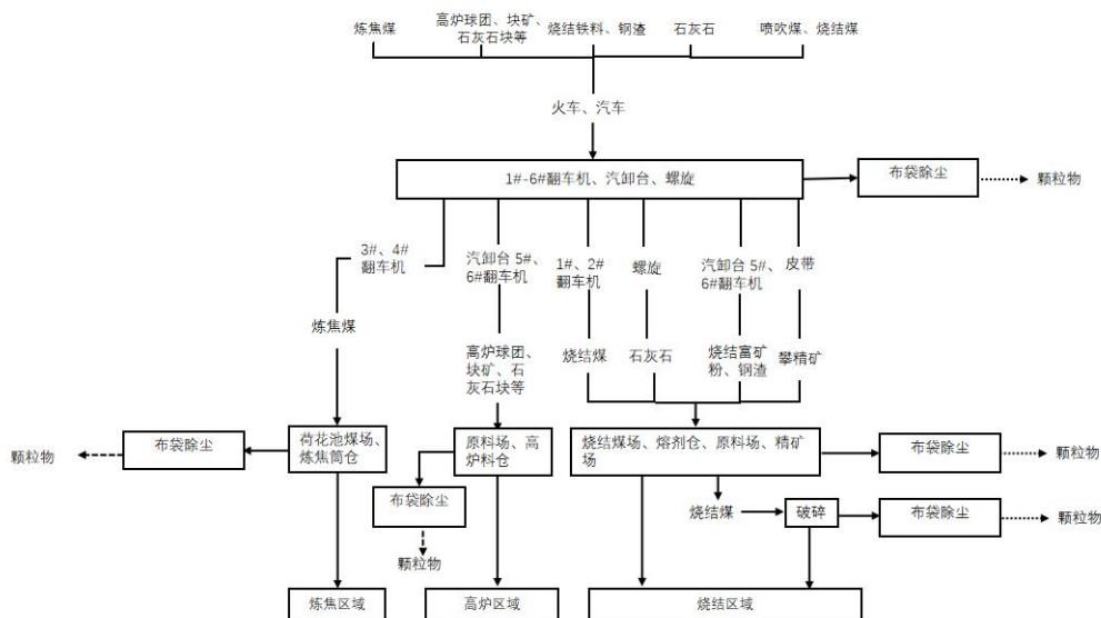
图 3-1 原料工序工艺流程及产排污图
