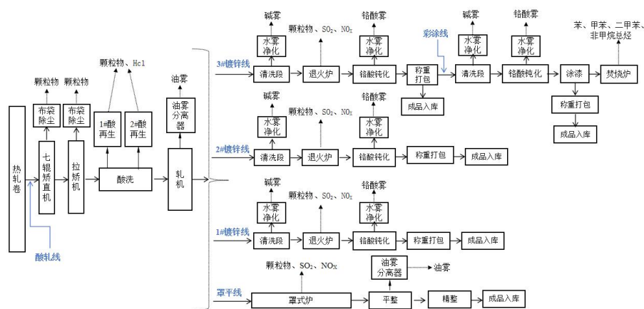
图 3-10 冷轧产排污节点工艺流程图
