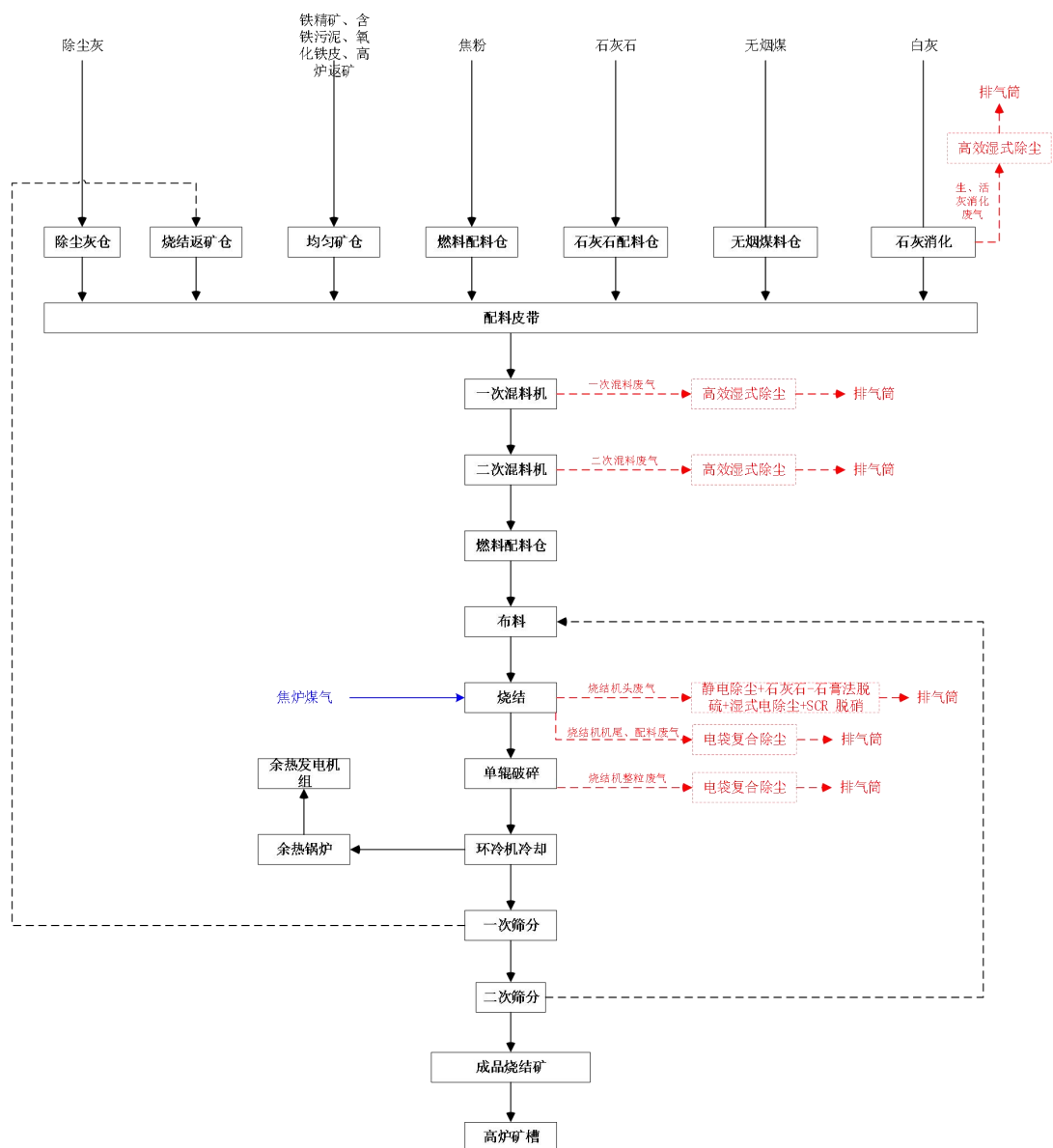
图 3-21 烧结装置工艺流程及产污环节图
