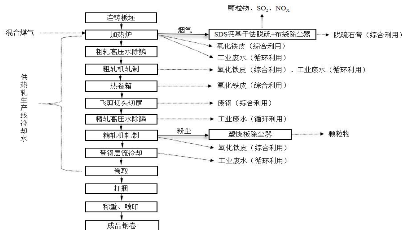
图 3-9 热轧产排污节点工艺流程图
