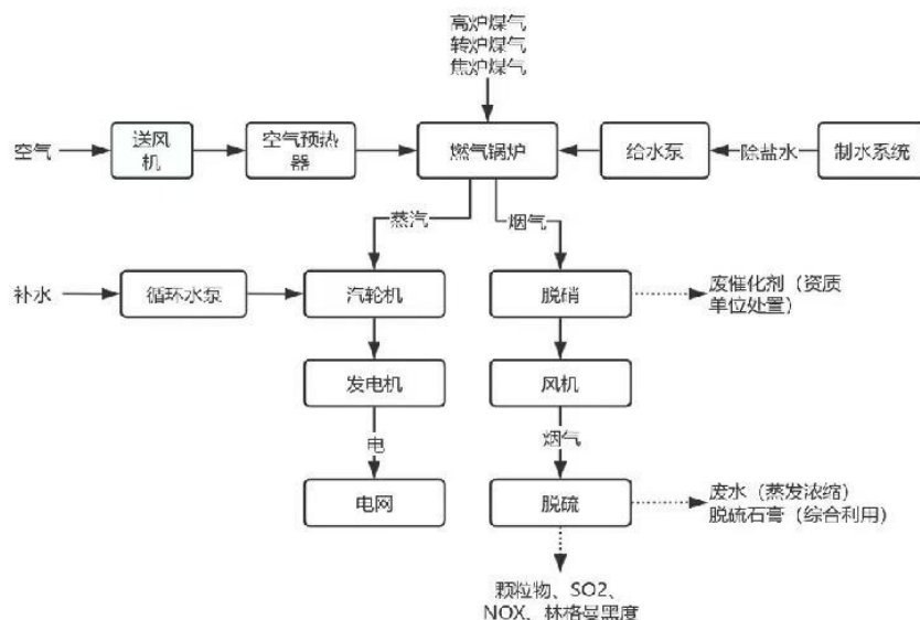
图 3-12 发电生产线工艺流程及产排污流程图
