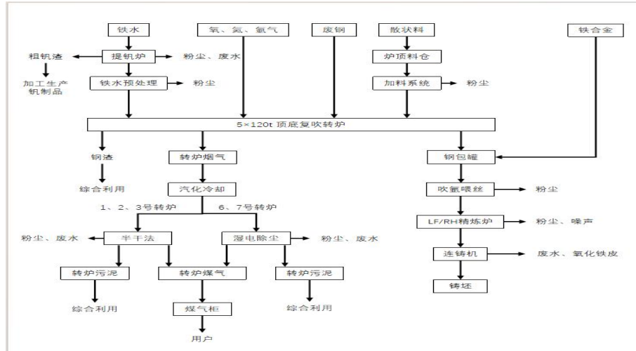
图 3-8 炼钢工艺流程及排污节点
