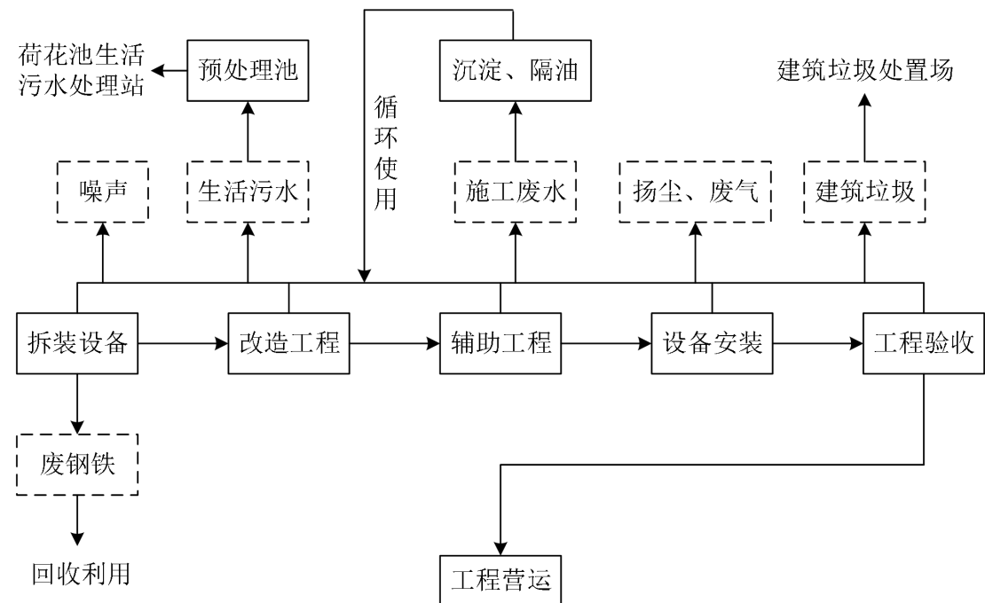
图 7-1 项目施工工艺流程及产污图
