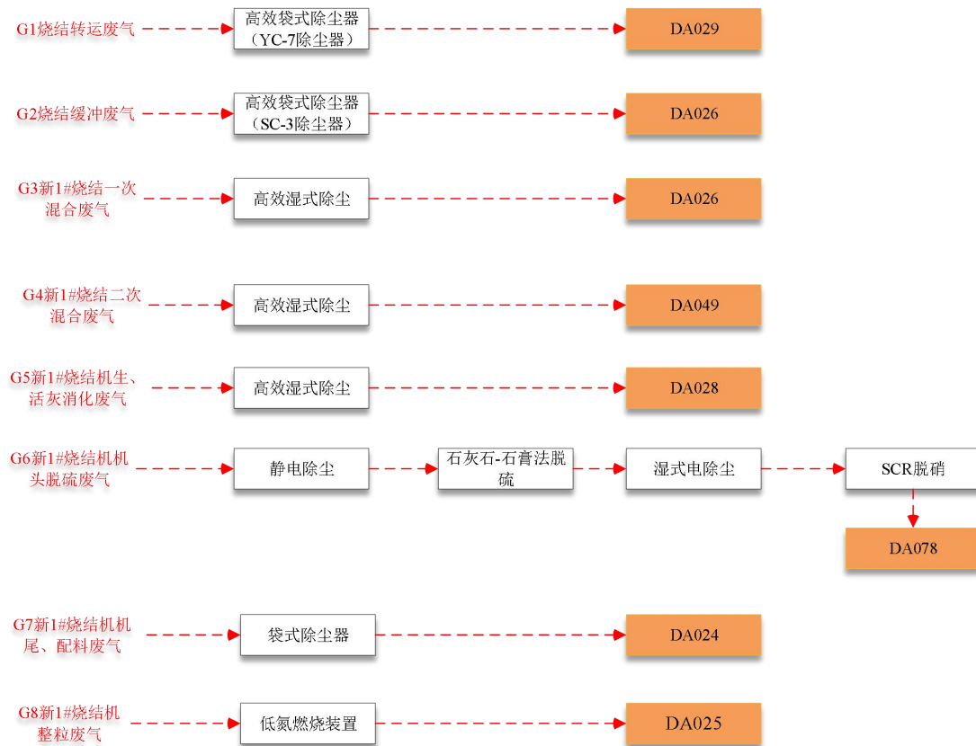
图 3-22 项目废气治理措施示意图
