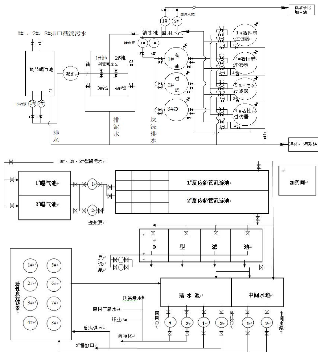
图 3-14 600m 3 污水处理系统工艺流程 荷花池污水处理系统工艺流程图
