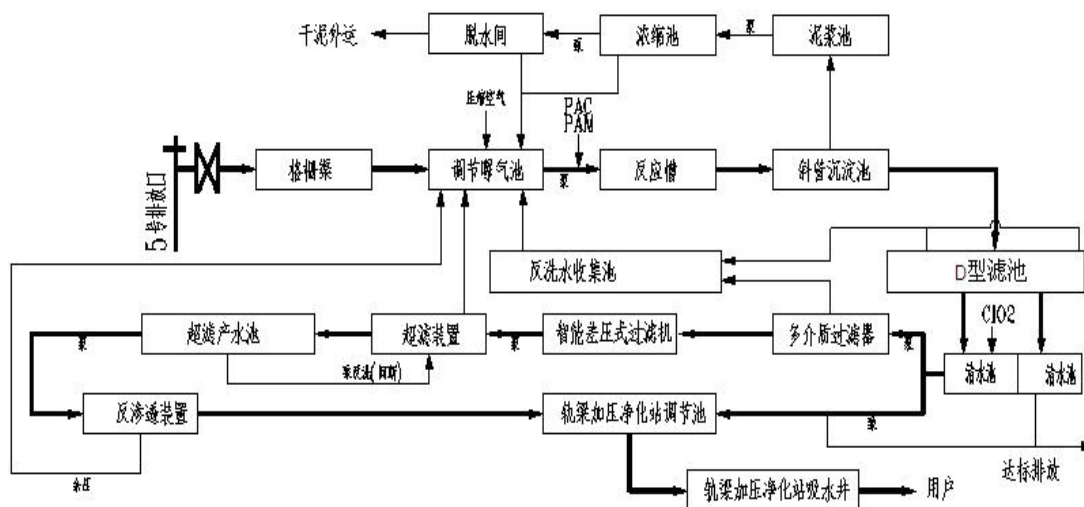
图 3-13 钢花污水处理系统工艺流程图
