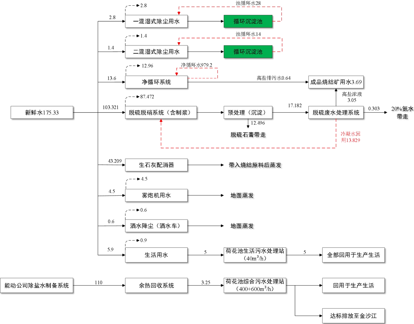
图 4-2 技改后烧结工序水平衡图 ( \text{m}^3/\text{d} )
