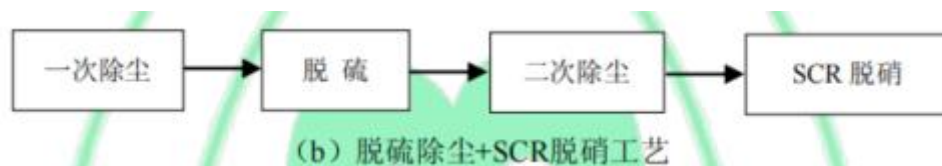
图 4-3 烧结机机头烟气超低排放典型工艺路线图
