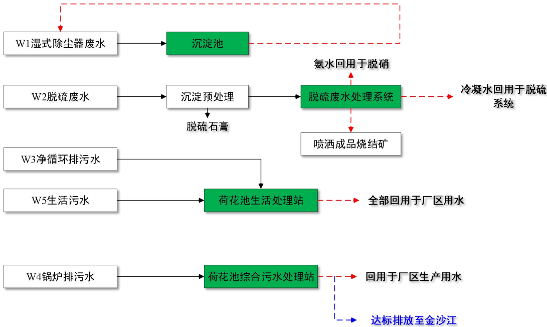
图 3-23 项目废水处理示意图
