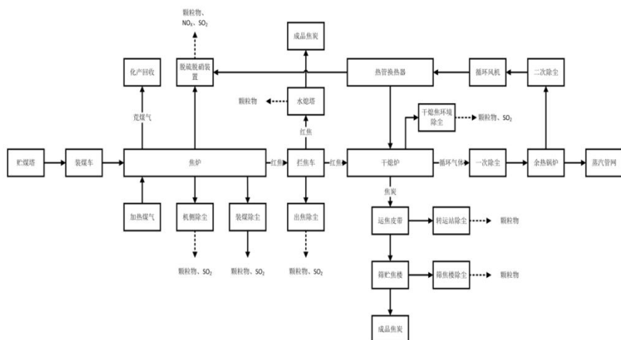
图 3-3 焦化工序 1、2 焦炉工艺流程及产排污图
