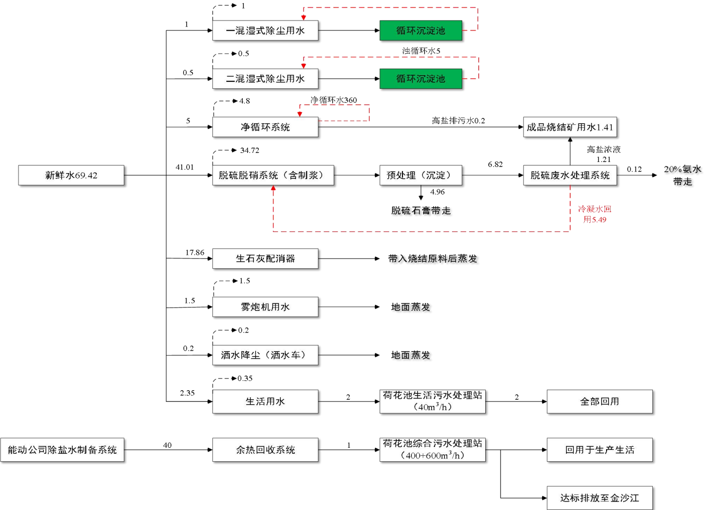
图 4-1 新 1#烧结机技改后水平衡图 (m³/h)
