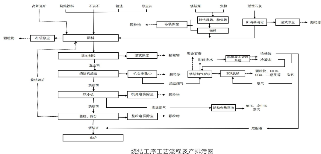
图 3-2 烧结工序工艺流程及产排污图
