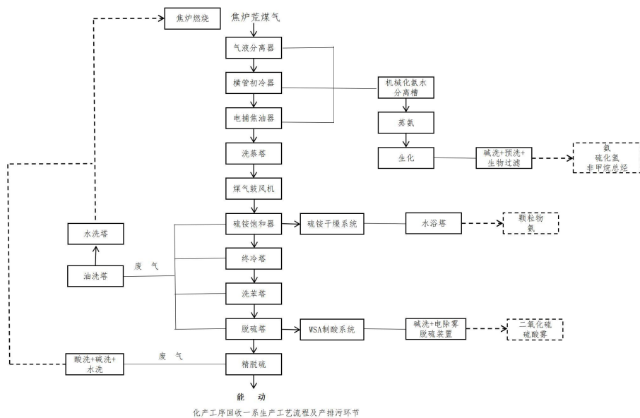
图 3-5 化产工序回收一系生产工艺流程及产排污图
