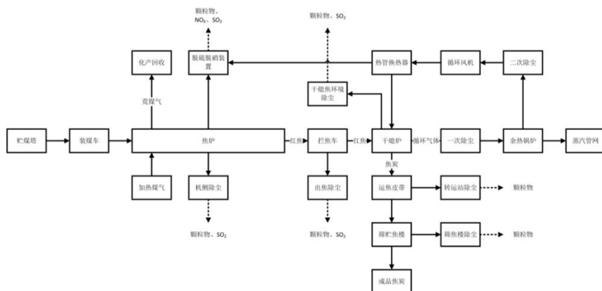
图 3-4 焦化工序 AB 焦炉工艺流程及产排污图
