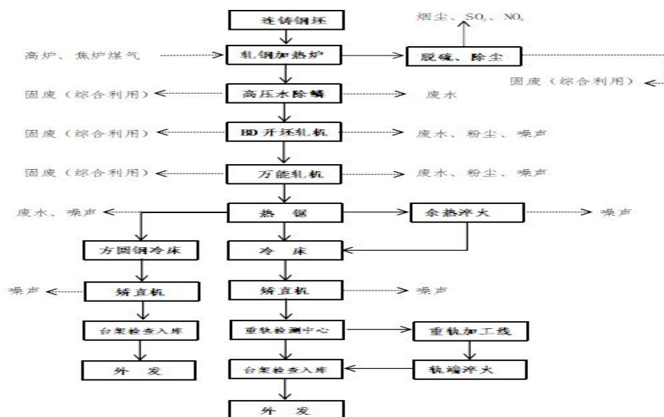
图 3-11 轨梁万能生产线工艺流程及产排污流程图
